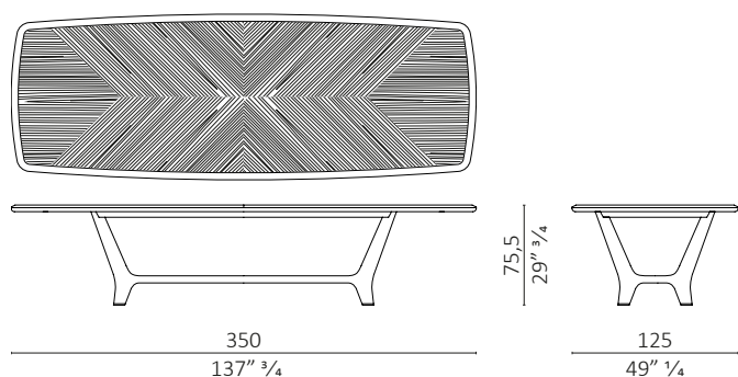
Grand Dîner rettangolare con top in legno / rectangular w wooden top
