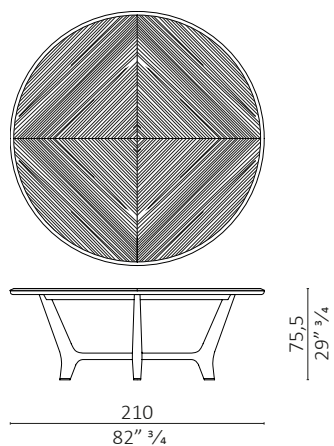
Grand Dîner ovale con top in legno / oval w wooden top
